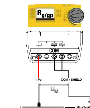
Messung: R_G Ableitwiderstand zu Schutzerde
