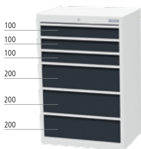
■ 6 x Tiroirs
