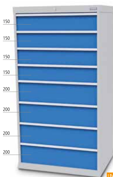
■ 8 x Tiroirs
