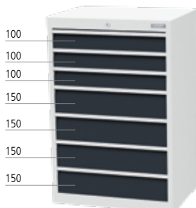
■ 7 x Tiroirs
