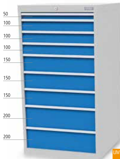
■ 9 x Tiroirs
