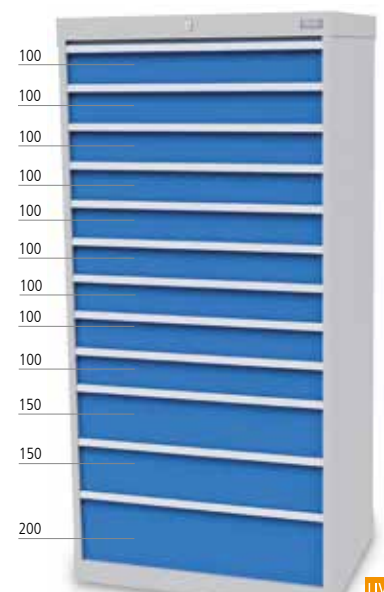
■ 12 x Tiroirs
