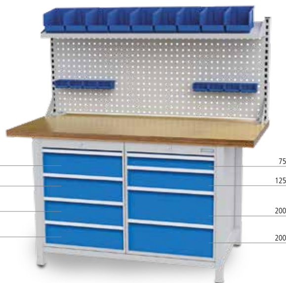
Kastenwerkbank R 18-24
