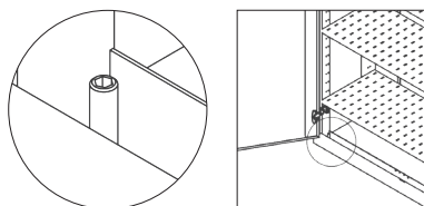
4 x Nivellierfüße von oben verstellbar mit einem Imbusschlüssel, Größe SW6
