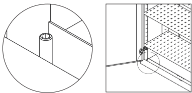
4 x Pieds de nivellement réglables par le haut à l'aide d'une clé hexagonale, taille SW6
