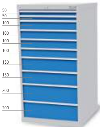
■ 10 x Schublade
