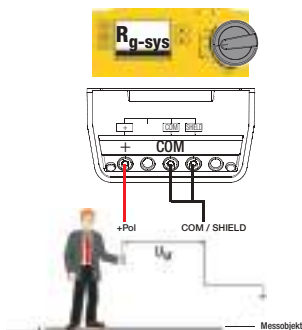
Messung: R_{g\text{-system}} Personenableitwiderstand (Mensch/Schuhe/Boden) zu Schutzerde
