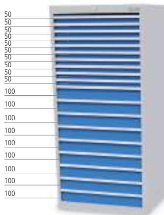
■ 19 x Schublade
