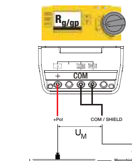
Messung: R_{g/gp} Ableitwiderstand zu Schutzerde
