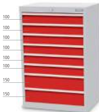
■ 8 x Schublade
