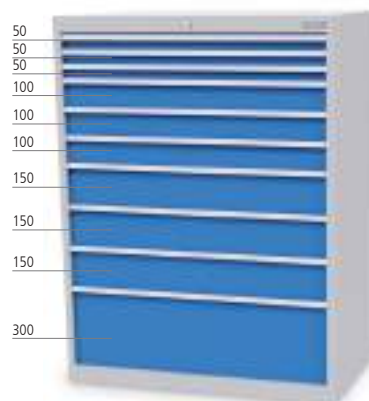
■ 10 x Schublade
