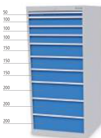
■ 10 x Schublade
