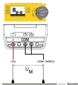
Messung: R_{p-p} Punkt-zu-Punkt Widerstand
