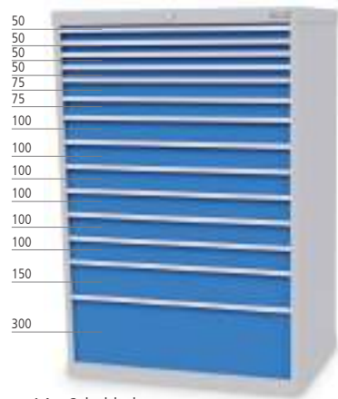
■ 14 x Schublade
